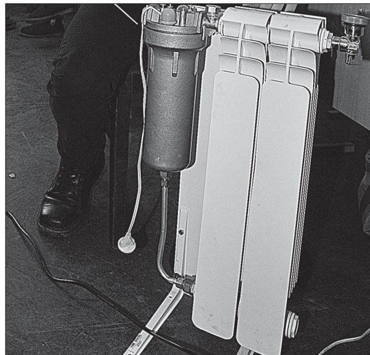
Павел Воцилин сделал компактный и экономный нагреватель для батарей. Теперь центральное отопление ему не нужно
