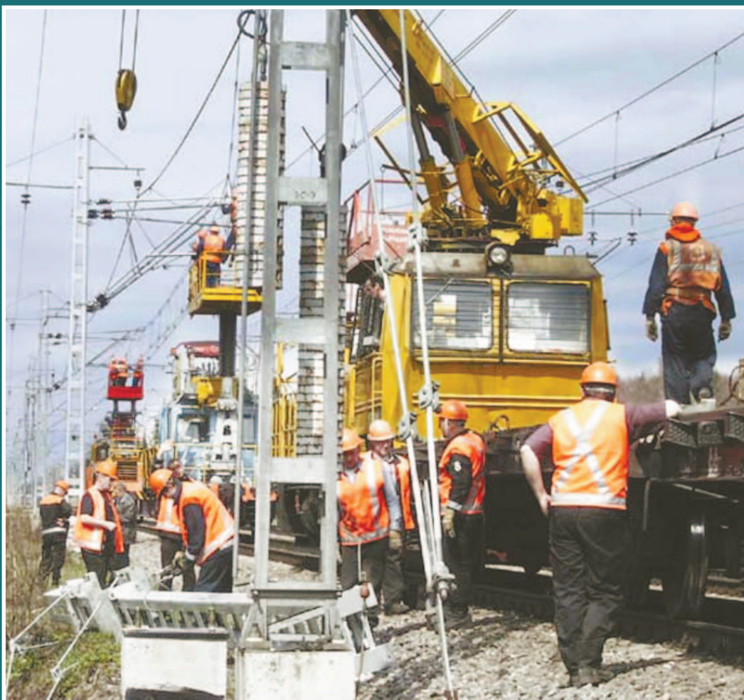
Монтаж опытных участков контактной сети для скорости движения 250 км/ч на участке Калашниково - Лихославль Октябрьской железной дороги
